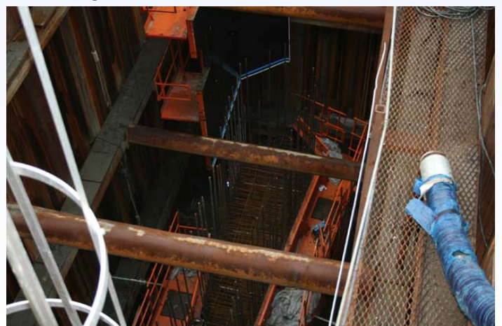
Encofrado en su sitio en la ataguía P7 alrededor de la jaula de armazón
