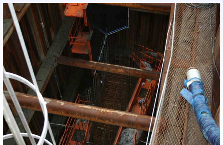
Cofragem no seu lugar no caixão P7 em volta da choldra de armação.
