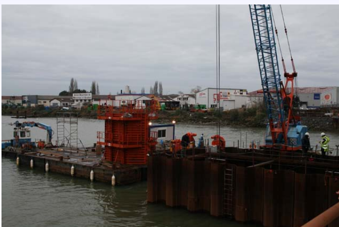
Operação de levantamento / cofragem no pilar P7
